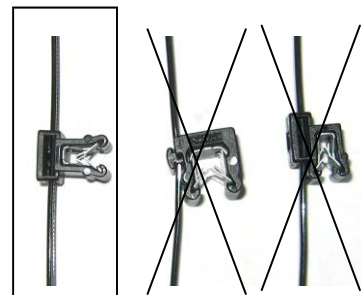
Edge Clips
